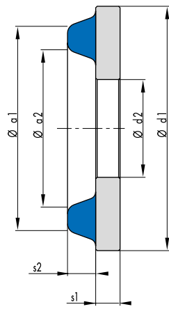
Abb. 2 Anschlagscheiben Typ I
