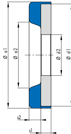
Abb. 3 Anschlagscheiben Typ II
