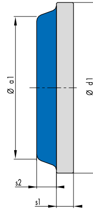
Abb. 4 Anschlagscheiben Typ III
