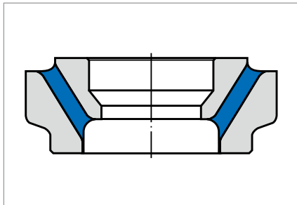
Abb. 1 Stützlager
