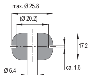
039 18 023 INSTRUMENTENHALTERUNG MIT TÜLLE
