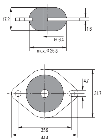
039 18 023 PLATTENFÖRMIGE INSTRUMENTENHALTERUNG
