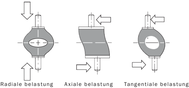
RICHTUNGSABHÄNGIGE BELASTUNG
