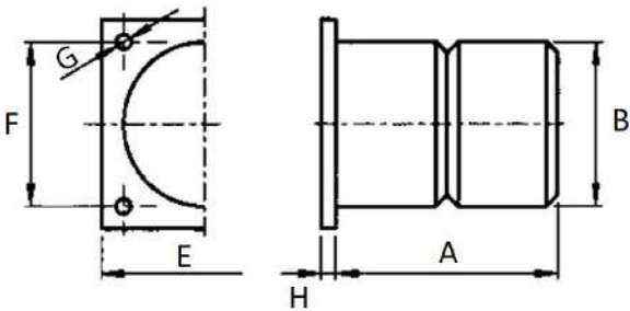
ZELLPUFFER MIT PLATTENBEFESTIGUNG
